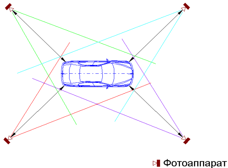
Рисунок. Схема выполнения фотосъемки транспортного средства (общего вида).
